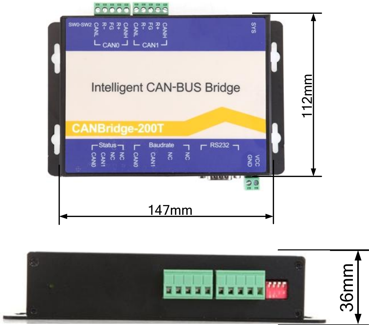
图 2-1-1 CANBridge-200T 智能CAN网桥机械尺寸
