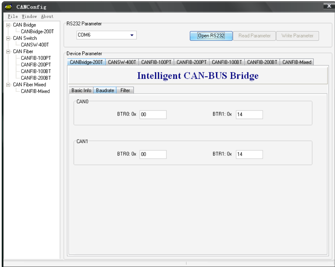
图 4-2-3-2-1 “Baudrate” 选项卡
