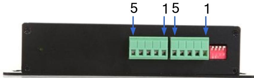
图2-2-2-1 CAN接线端子
