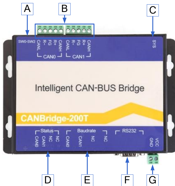
图 2-2-1-1 设备接口
